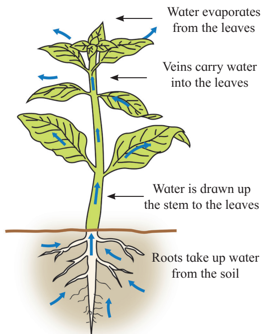
Fig. 6.6 : Transpiration
